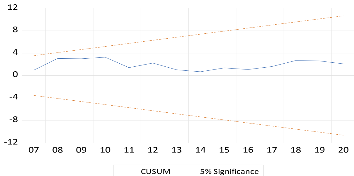
Fig. 6. CUSUM test
